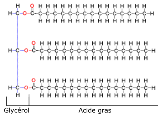
Figure 1 : Triglycéride
